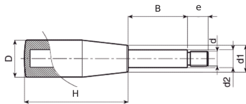
Espiga roscada de acero cincado. Mango cilíndrico de poliamida negra reforzada.
