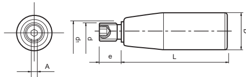
Espiga de acero cincado. PA: Poliamida negra reforzada.
